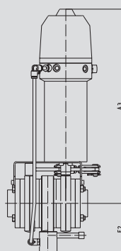
leakage b.v. LSV07 1LV inch BF PAMS + TOP item-no. 59641-
